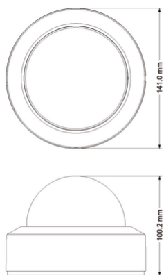
Vista ingombri
