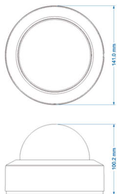
Vista ingombri
