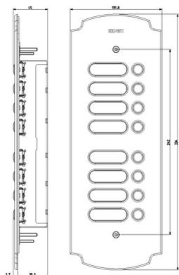
Vista ingombri
