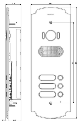
Vista ingombri
