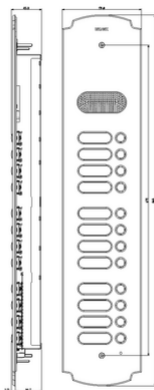
Vista ingombri
