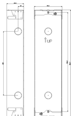
Vista ingombri
