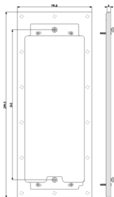
Vista ingombri
