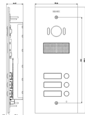
Vista ingombri
