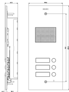
Vista ingombri
