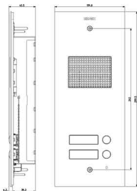
Vista ingombri
