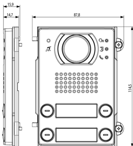
Vista ingombri
