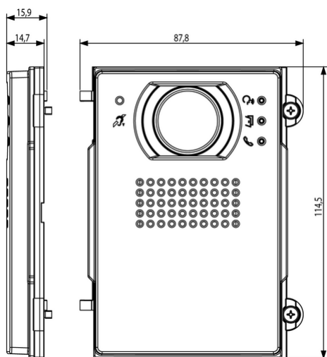
Vista ingombri
