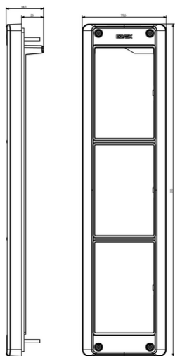
Vista ingombri
