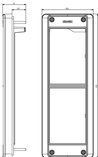
Vista ingombri
