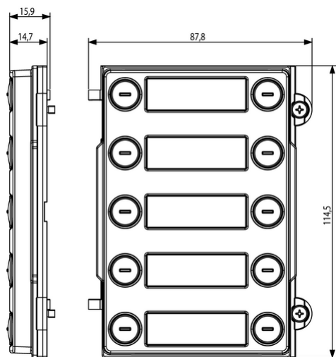
Vista ingombri
