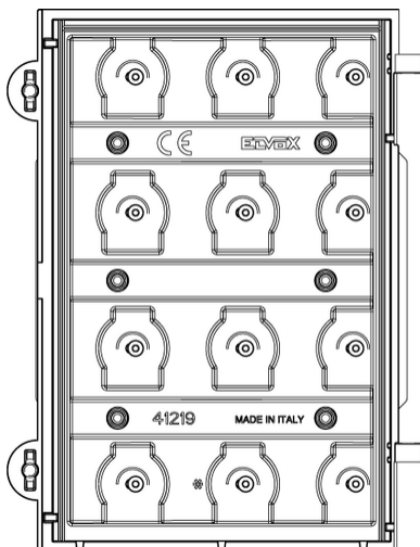
Vista posteriore
