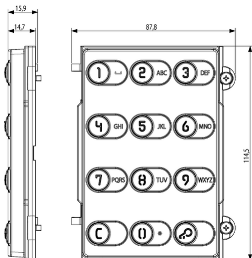
Vista ingombri
