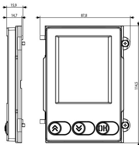
Vista ingombri
