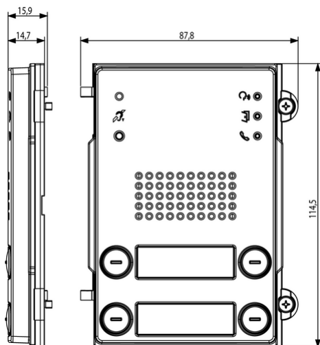
Vista ingombri
