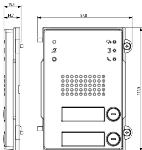
Vista ingombri
