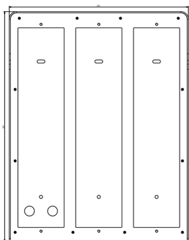
Vista ingombri
