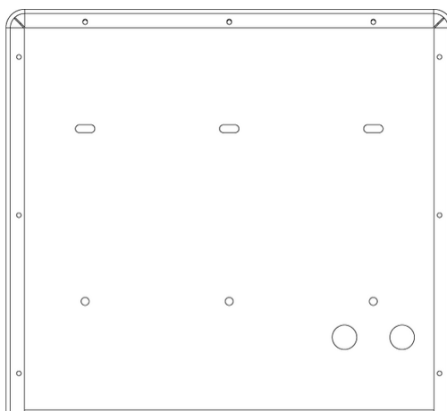
Vista posteriore
