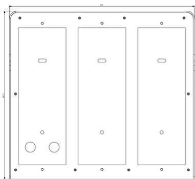
Vista ingombri
