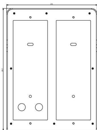
Vista ingombri
