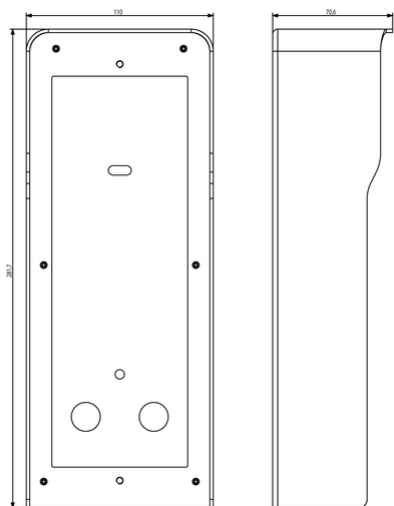
Vista ingombri
