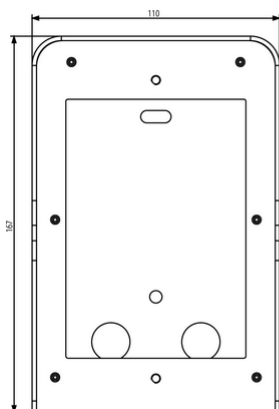
Vista ingombri
