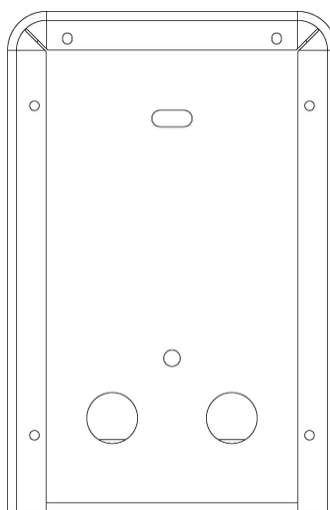
Vista posteriore
