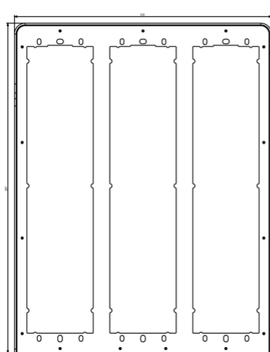
Vista ingombri
