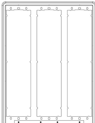
Vista posteriore
