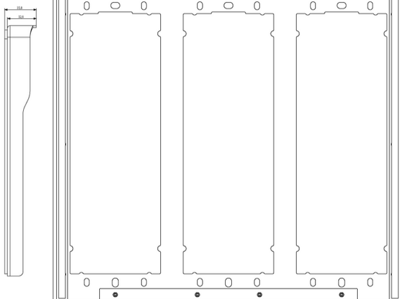
Vista posteriore
