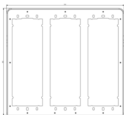
Vista ingombri
