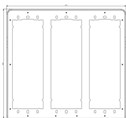
Vista ingombri
