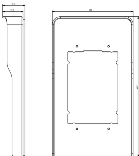
Vista ingombri
