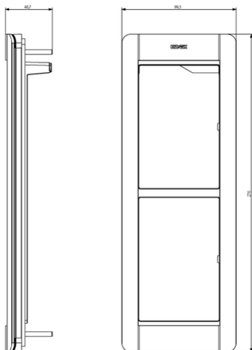
Vista ingombri
