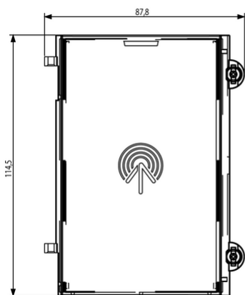
Vista ingombri
