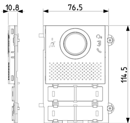
Vista ingombri
