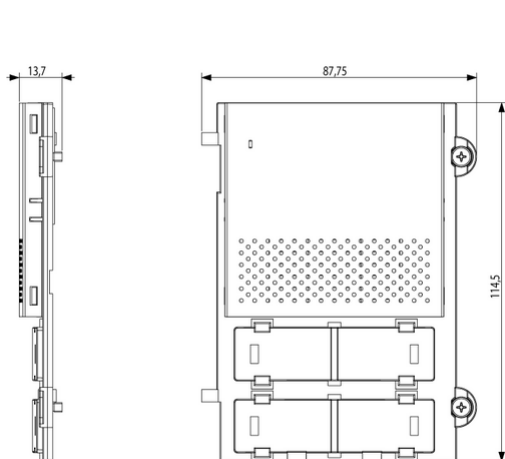
Vista ingombri
