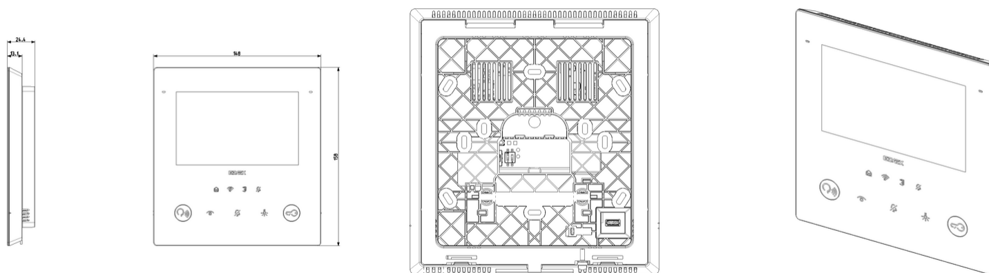
Vista ingombri
