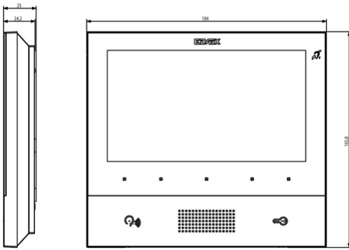
Vista ingombri
