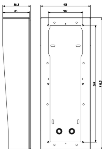
Vista ingombri
