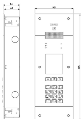
Vista ingombri
