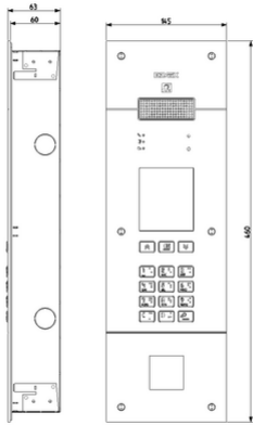
Vista ingombri
