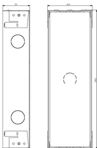
Vista ingombri
