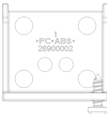
Vista posteriore
