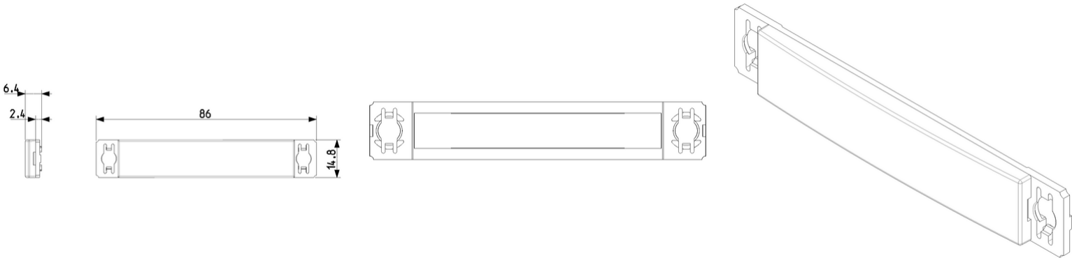
Vista ingombri
