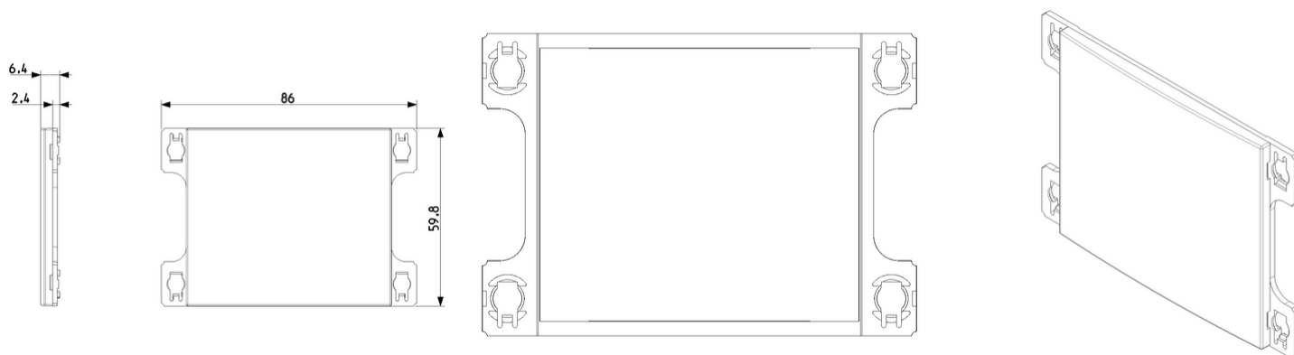
Vista ingombri
