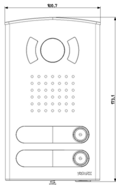
Vista ingombri
