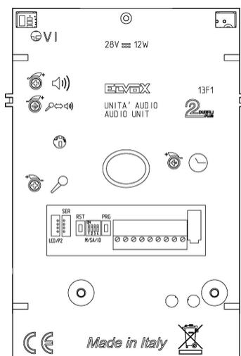
Vista posteriore
