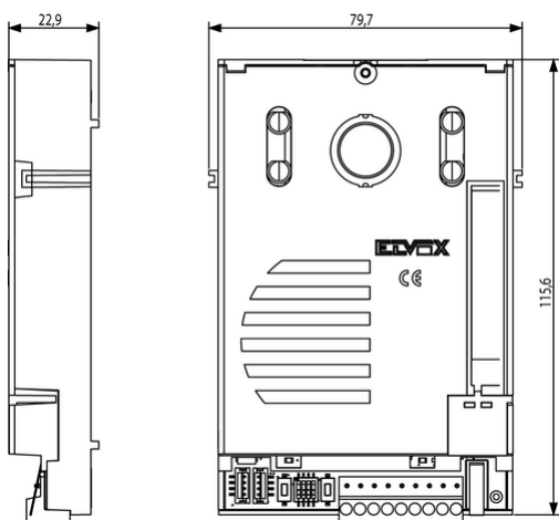
Vista ingombri
