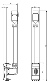
Vista ingombri
