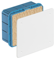
V70005 - Scatola derivazione incasso 154x128x70mm
