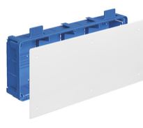
V72008 - Scatola deriv. p/leggere 402x164x73,5mm
