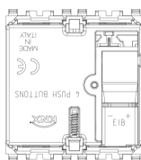
Vista posteriore
