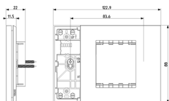
Vista ingombri
