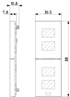
Vista ingombri
