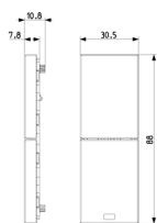
Vista ingombri
